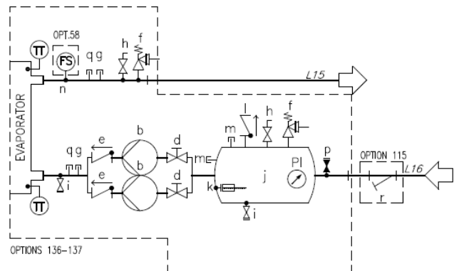
Рис. 9. Гидравлическая схема для двояного насоса (EWYTx5B) (компл. 80-81/136-137) (макс. рабочее давление 6 бар)
