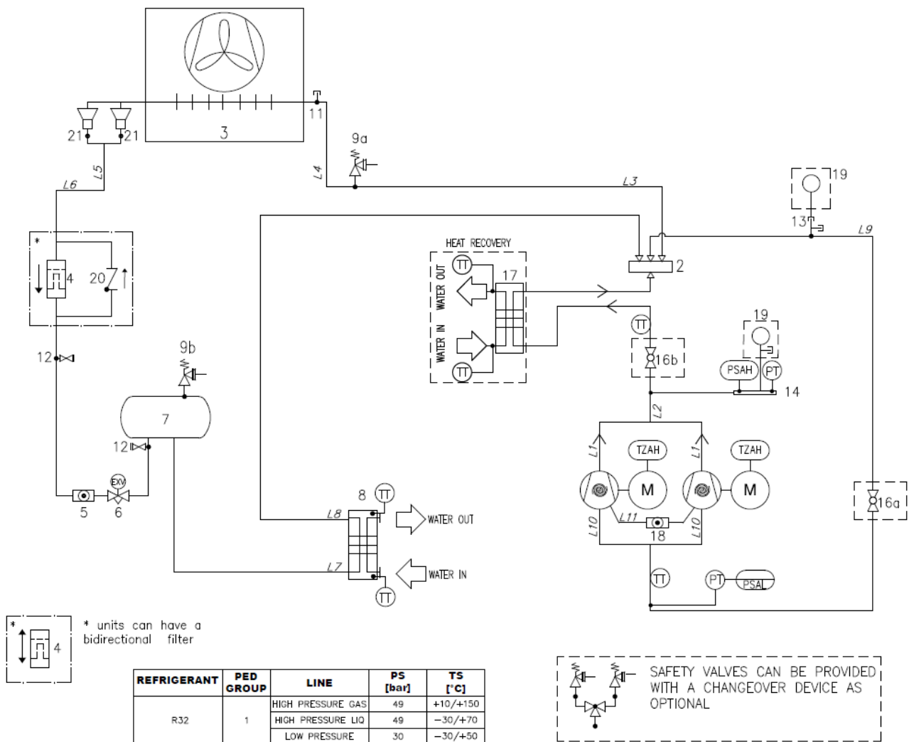
Рис. 19. Схема трубопровода хладагента (схема трубопроводов и КИП) для одноконтурного агрегата EWYTxx5B
