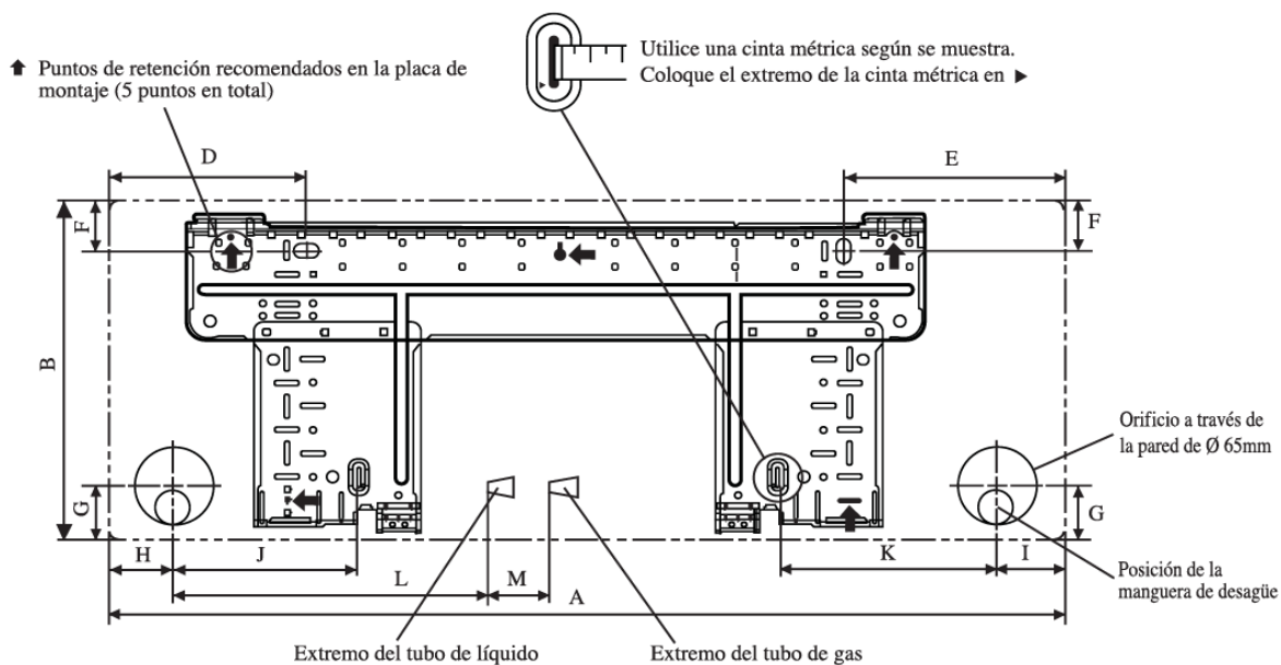
PLACA DE INSTALACIÓN 20/25/35
