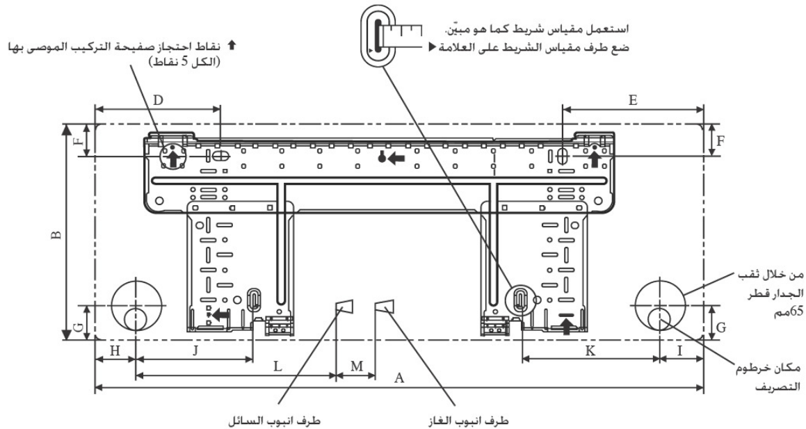
لوحة التركيب 25/35
