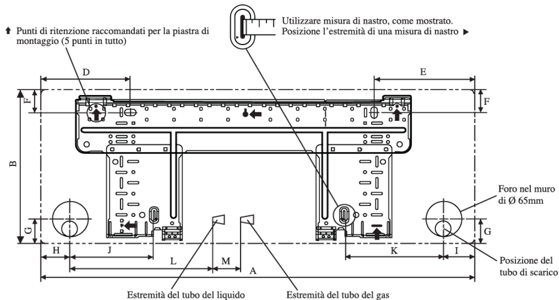
LASTRA DI INSTALLAZIONE 20/25/35
