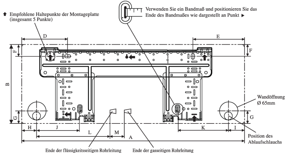
MONTAGEPLATTE 20/25/35
