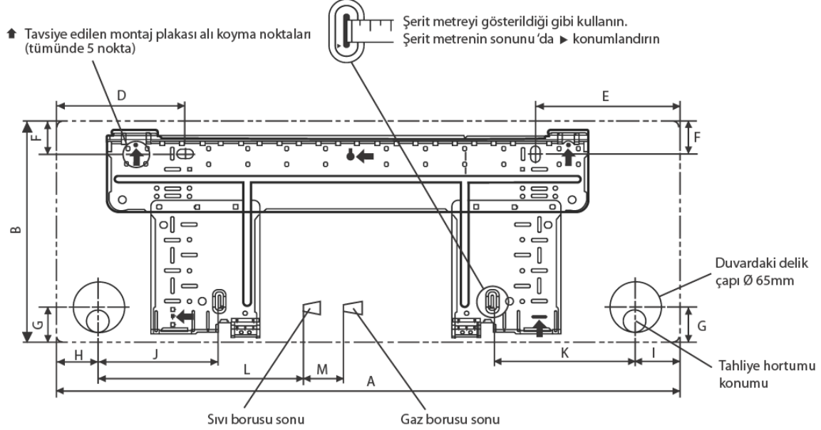
KURULUM LEVHASI 20/25/35
