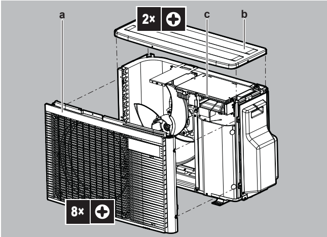
a Лицевая панель b Верхняя панель c Разъем S99
